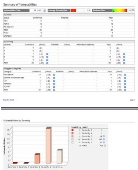
Schéma 8 : Rapport « Executif »
